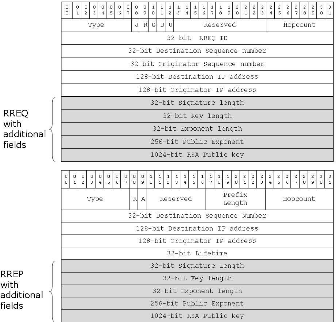
Fig. 1. SecAODV Message Formats
